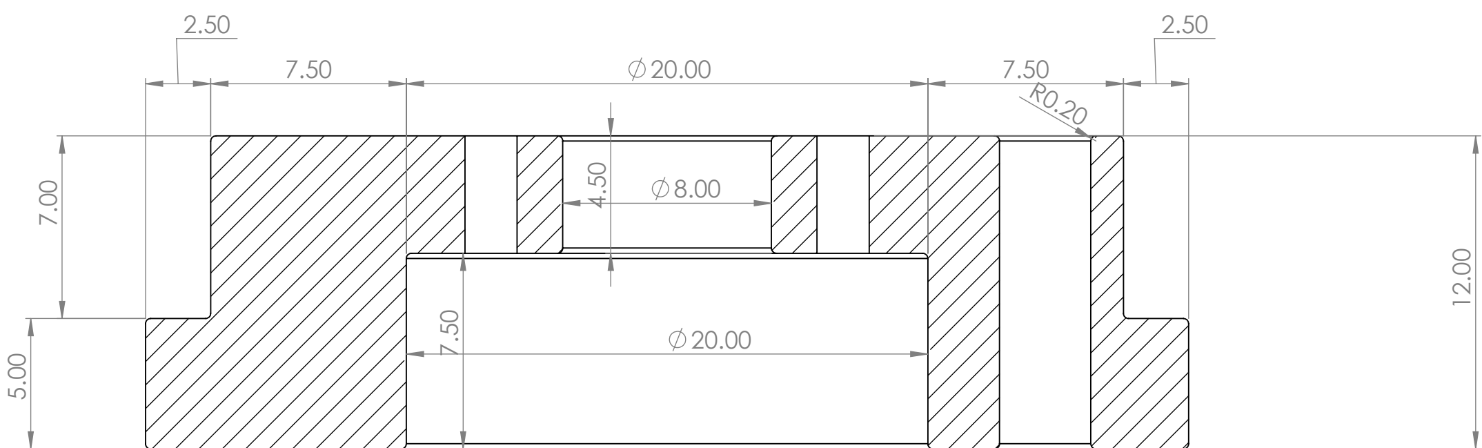
SECTION A-A
